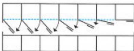
Stalschema met wegdraaibare voorwanden
